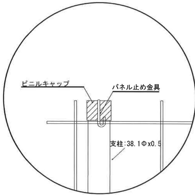
あ部 詳細図
